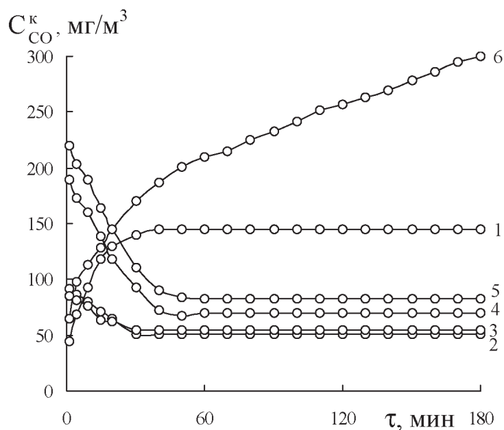
Рис. 2. Изменение C_{CO}^k во времени при окислении CO кислородом в присутствии образцов 1–6 катализатора K_2PdCl_4-Cu(NO_3)_2-H_2O/Н-Кл-6 . Последовательность стадии и условия приготовления катализатора представлены в табл. 2
