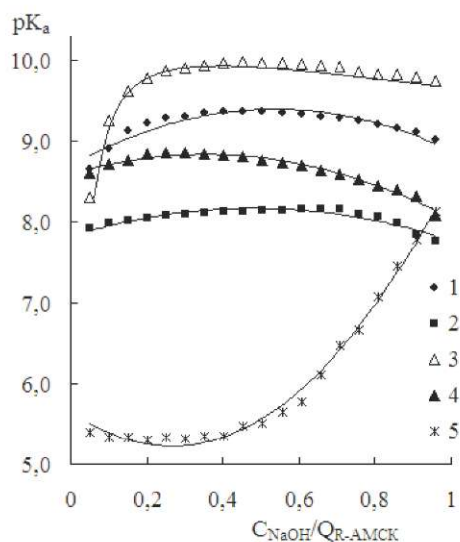
Рис. 3. Концентрационные зависимости pK_a в системах R-AMСК – NaOH – H 2 O. R-AMСК: I – 1; II – 2; III – 3; IV – 4; V – 5.
