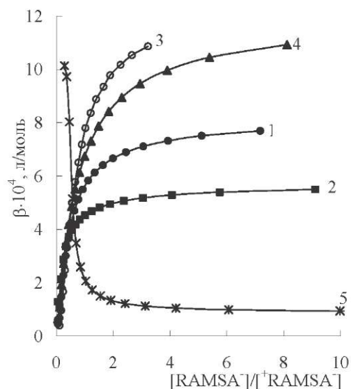
Рис. 4. Зависимость буферной емкости ( \beta ) растворов R-AMCK – NaOH – H 2 O от соотношения
