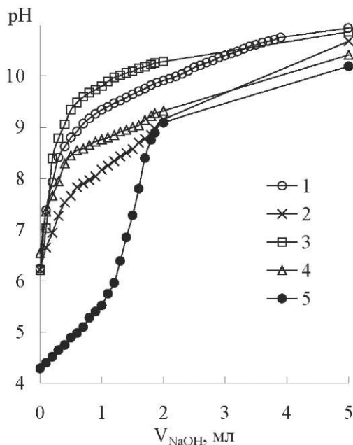
Рис. 1. рН-метрические кривые титрования водных растворов N-производных АМСК водным раствором NaOH. V_{R-AMSK}^0 = 20 мл C_{R-AMSK}^0 = 0,001 М; C_{NaOH}^0 = 0,01 М. R-АМСК: I - 1; II - 2; III - 3; IV - 4; V - 5.
