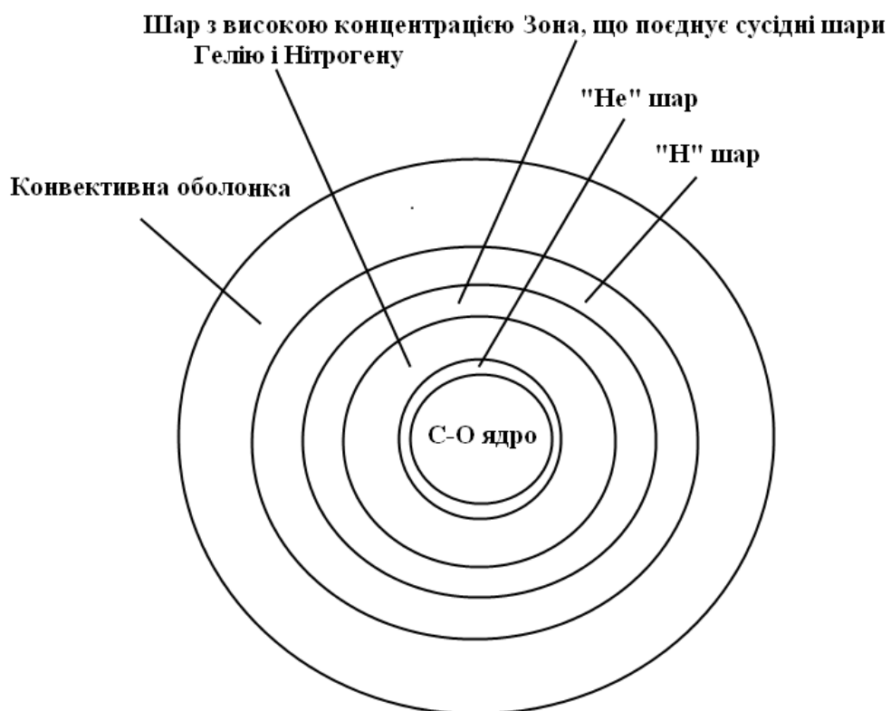
Рис. 7. Структура зорі асимптотичної гілки гігантів
