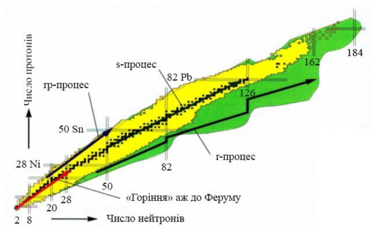
Рис. 15. Діаграма нуклідів у координатах заряд ядра–число нейтронів із вказівкою процесів їх утворення
