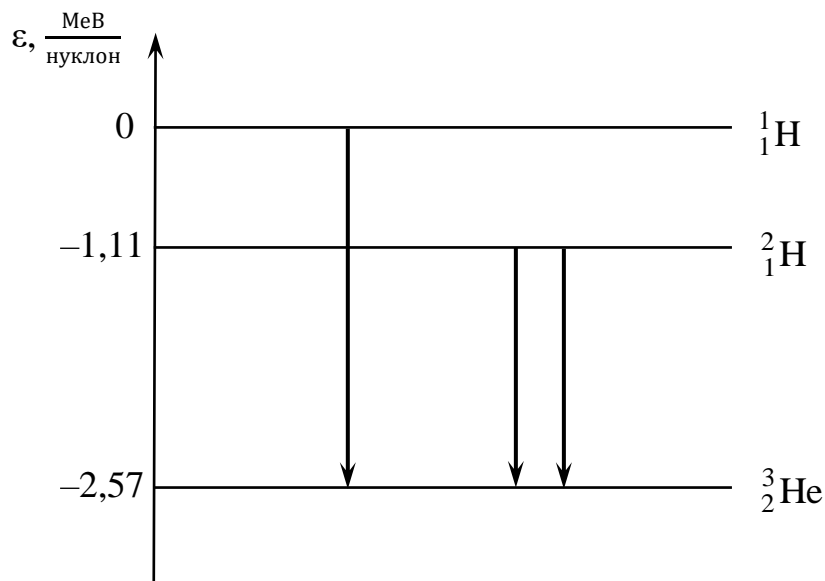
Рис. 2. Енергетична діаграма переходів нуклонів у реакції синтезу ядра легкого ізоотопу Гелію ( {}^3_2\text{He} )
