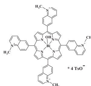
Ві(III)-мезо-тетра(6-N-метил-хінолініл)порфірин
