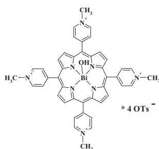
Ві(III)-мезо-тетра(4-N-метил-піридил)порфірин
