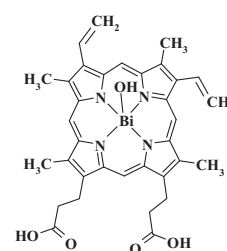
Ві(III)-протопорфірин IX
