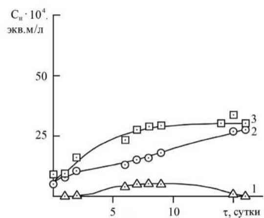
Рис. 3. Зависимость концентрации ионов от времени выщелачивания для системы отвал + 0,1n H 2 SO 4 . Сн, экв.м./л: 1 – Fe 2+ , 2 – Fe 3+ , 3 – Fe общ .
