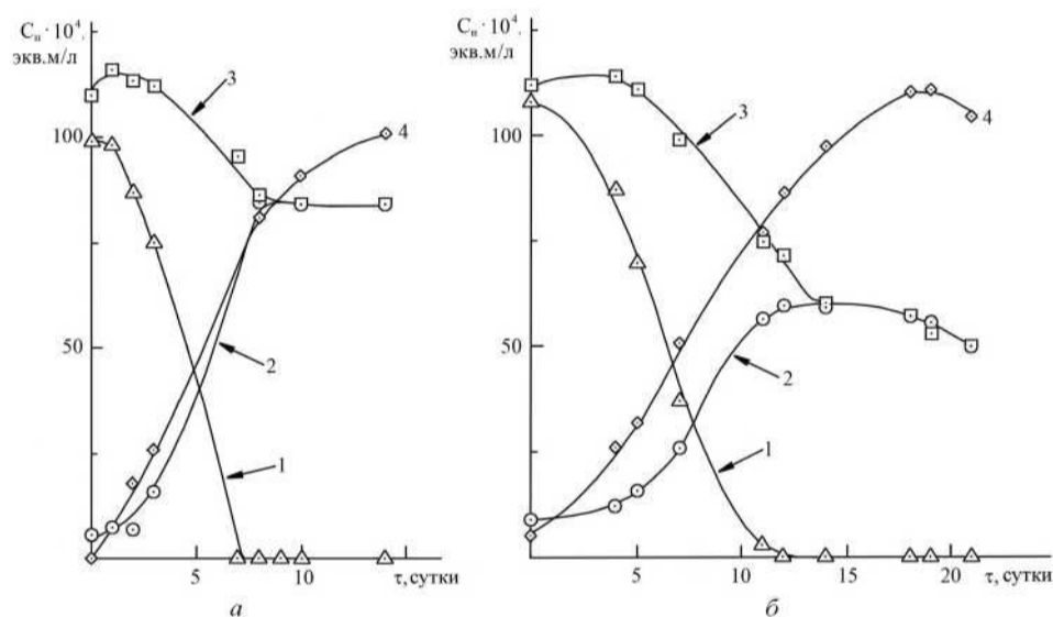
Рис. 4. Зависимость концентрации ионов от времени выщелачивания для системы отвал + питательная среда без штаммов бактерий ( а) и в их присутствии (б). Сн, экв.м./л: 1 – Fe 2+ , 2 – Fe 3+ , 3 – Fe общ , 4 – Me Y+ .
