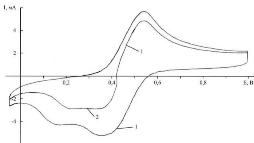
Рис. 1. Циклические I-E кривые при разворачивании потенциала в анодную (1) и катодную (2) области для системы отвал + питательная среда. Условия съемки: v_{раз} = 20 мВ/с; x = 50 мВ/см; y = 1 мА/см
