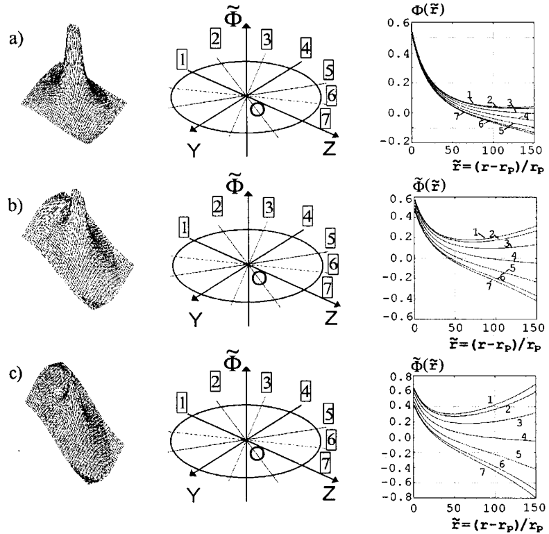
Рис. 3. Розподіл самоузгодженого електростатичного потенціалу в чарунці електронейтральності C_{\xi}^z гетерогенної плазмової системи зі стаціонарним струмом в об'ємі, поляризованої зовнішнім електростатичним полем. Напрямки 1...7 утворюють рівномірну сітку за кутом \theta між \vec{E}_0 та радіус вектором \vec{r} з вузлами: \left\{ \pi, \frac{5}{6}\pi, \frac{2}{3}\pi, \frac{1}{2}\pi, \frac{1}{3}\pi, \frac{1}{6}\pi, 0 \right\} ; модуль напруженості зовнішнього електричного поля у випадках а), б), в) відповідно складає: |\vec{E}_0| = 0.1 \cdot |\Phi_Q|, 0.3 \cdot |\Phi_Q|, 0.5 \cdot |\Phi_Q| ; \Phi_Q = ze^2 / (r_p^2 \cdot kT) – кулонівське поле КЧ
