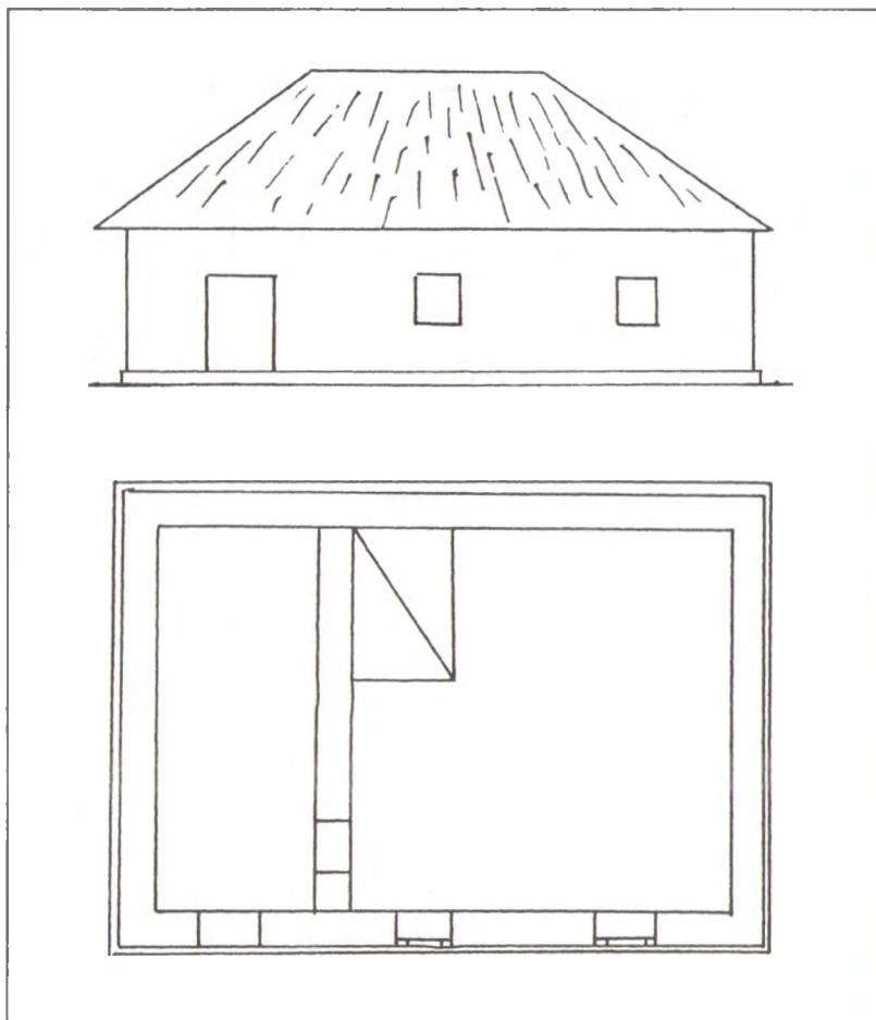
Мал. 5. 1 — План будинка для однієї родини
