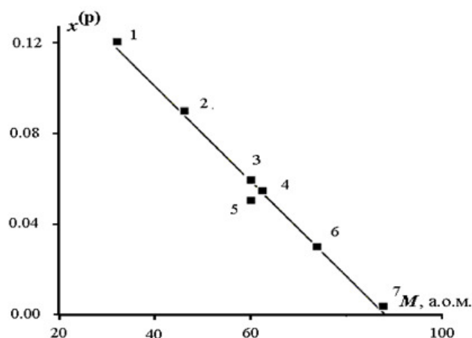
Рис. 1. Залежність координат особливої точки розчинів спиртів x^{(p)} [7], визначені за аномальним розсіянням світла, від молекулярної маси розчинених спиртів: 1 – метанол; 2 – етанол; 4 – етіленгліколь; 6 – третинний бутанол; 7 – пентанол. В центрі кривої точки відповідають ізомерам: 5 – н-пропанол (пропиловий спирт, 1 – пропанол) та 3 – ізопропанол (2-пропанол).
