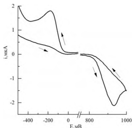
Рис. 1. Циклическая вольтамперограмма раствора КАН на фоне универсального буферного раствора с pH 2; скорость развертки потенциала 50 мВ/с; C_{\text{KAN}}=1 \cdot 10^{-4} моль/л
