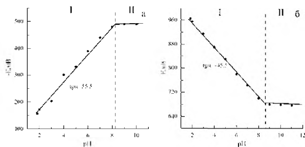
Рис. 4. Влияние pH среды на потенциалы пиков: а) восстановления; б) окисления кармоазина в водных растворах
