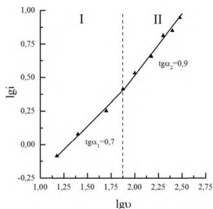
Рис. 2. Определение величины критерия Семерано для процесса восстановления КАН; C_{\text{KAN}}=1 \cdot 10^{-4} моль/л; фоновый электролит — универсальный буферный раствор с pH 2
