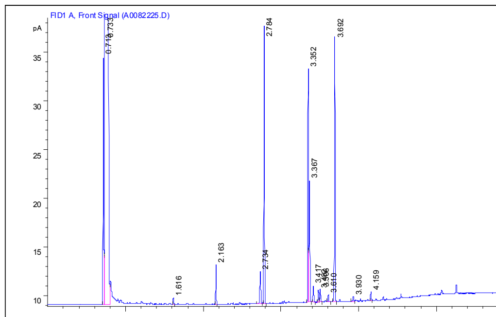
Рис. 5. Хроматограма спектру ефірів жирних кислот бактерій штаму L. bifermentans 19
