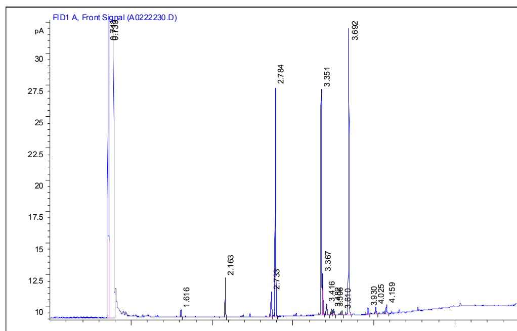
Рис. 6. Хромотограма спектру ефірів жирних кислот бактерій штаму L. vaccinostercus 22
