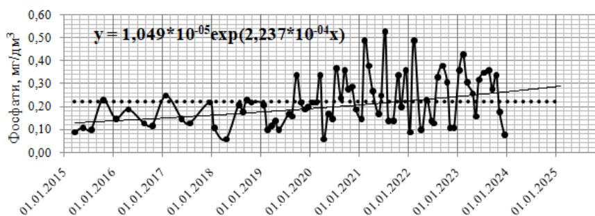
Рис. 1 – Хронологічна мінливість показника PO_4^{3-} (р. Дунай, м. Кілія) Fig. 1 - Chronological variability of the PO_4^{3-} indicator (Danube River, Kiliya town)
