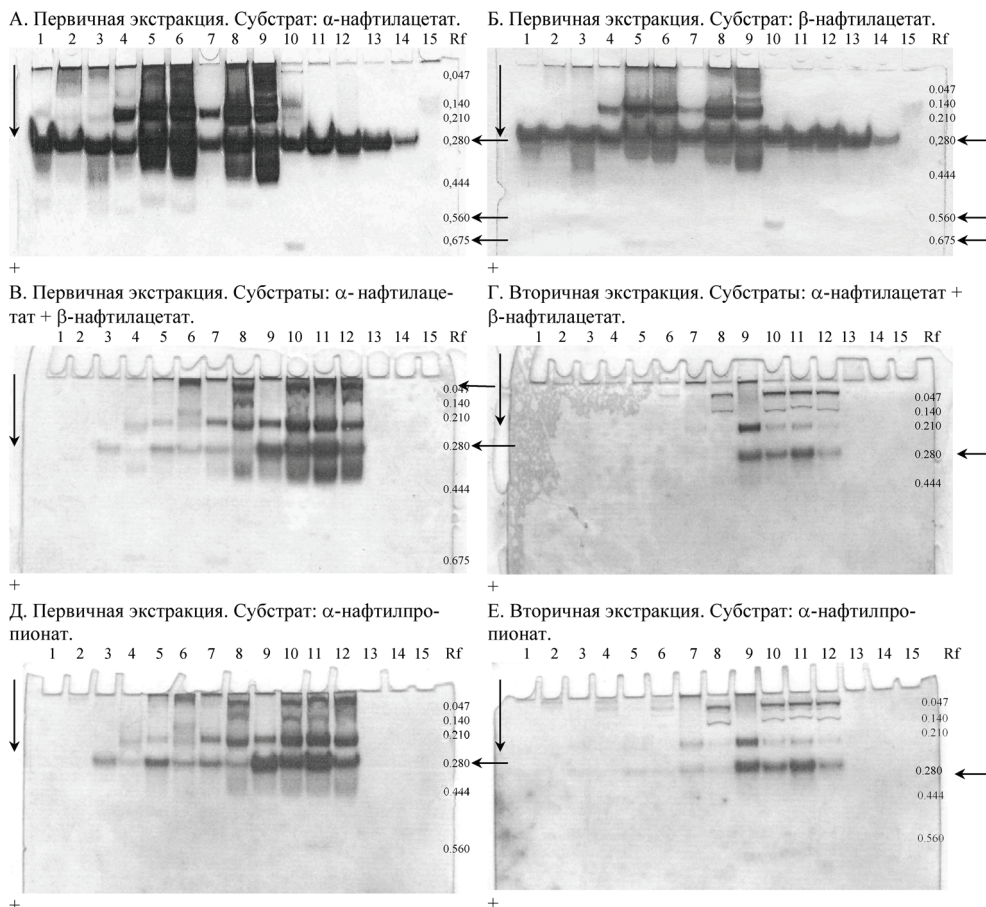
Рис. 1. Спектры гидролаз эфиров карбоновых кислот в онтогенезе Drosophila melanogaster :
