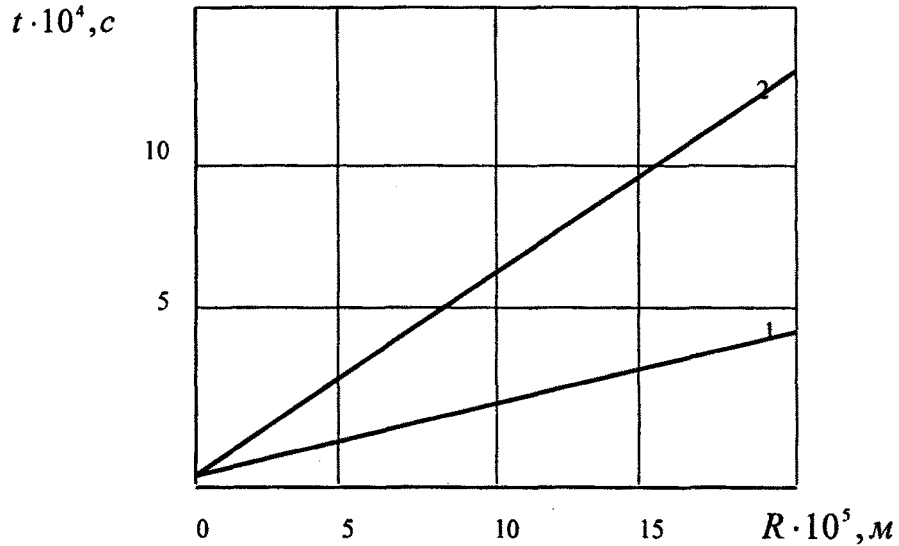
Рис.4. Зависимость времени процессов от первоначального размера капли R : 1– время растягивания капли в струю t_k , 2– полное время взаимодействия капель при частичном слиянии t_n
