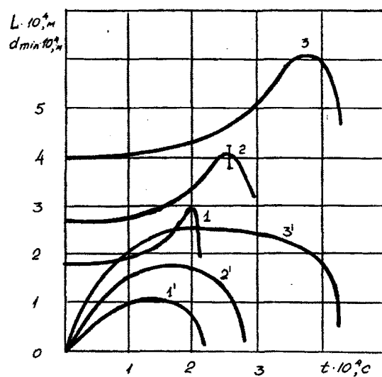
Рис.6. Кинетика развития струи растяжения: 1,2,3– зависимости длины струи L(t) , 1',2',3'– зависимости d(t) , R=88 мкм; 130 мкм; 200 мкм соответственно, \alpha=35^\circ , v_1=1,2+1,4 м/с
