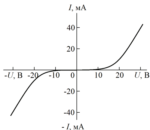
Рис.1. Вольт-амперная характеристика варистора на основе SiC.
