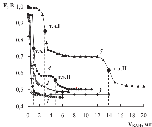
Рис. 4. Редокс-метрическое титрование системы «Mn(VII)–Cr(VI)» водным раствором КАН (pH 2): 1–Mn:Cr=1:1, 2–Mn:Cr=1:5, 3 –Mn:Cr=1:10, 4 –Mn:Cr=5:1, 5 –Mn:Cr=10:1. C_M = C_{КАН} = 1 \cdot 10^{-3} моль/дм 3 .
