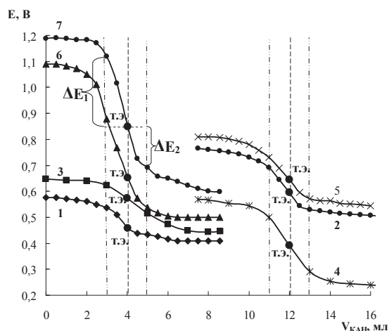
Рис. 1. Кривые редокс-метрического титрования ионов металлов водным раствором КАН: 1– \text{Hg(II)} ; 2– \text{Cr(VI)} ; 3– \text{Mn(VII)} , pH 6,0; 4– \text{Se(VI)} ; 5– \text{V(V)} ; 6– \text{Mn(VII)} , pH 2,0; 7– \text{Ce(IV)} .
