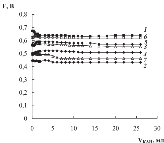
Рис. 3. Редокс-метрическое титрование системы «V(V)–Se(VI)» водным раствором КАН (рН 0): 1–V(V), 2–Se(VI), 3–V:Se=1:1, 4–V:Se=5:1, 5–V:Se=1:5, 6–V:Se=10:1, 7–V:Se=1:10. C_M = C_{\text{КАН}} = 1 \cdot 10^{-3} моль/дм 3 .
