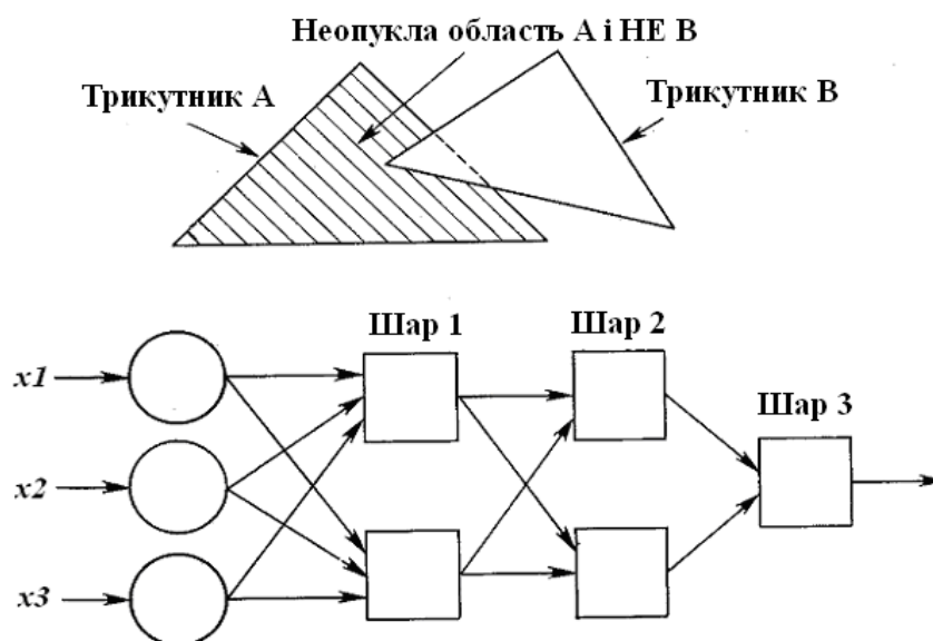
Рис. 3.12 – Увігнута область рішень, що задається тришаровою мережею
