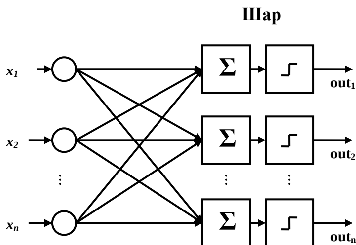
Рис. 3.3 – Архітектура одношарового персептрона з багатьма виходами
