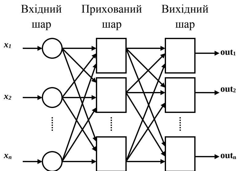
Рис. 3.6 – Архітектура багатошарового (двошарового) персептрона
