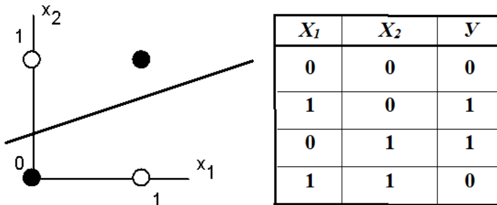
Рис. 3.4 – Проблема «що виключає АБО» одношарового персептрона (білі точки не можуть бути відокремлені однією прямою від чорних)
