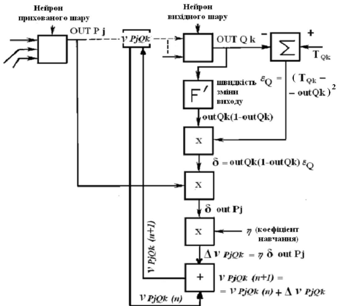
Рис. 3.8 – Підстроювання ваг вихідного шару
