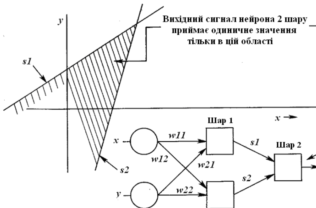
Рис. 3.11 – Опукла область рішень, що задається двошаровою мережею
