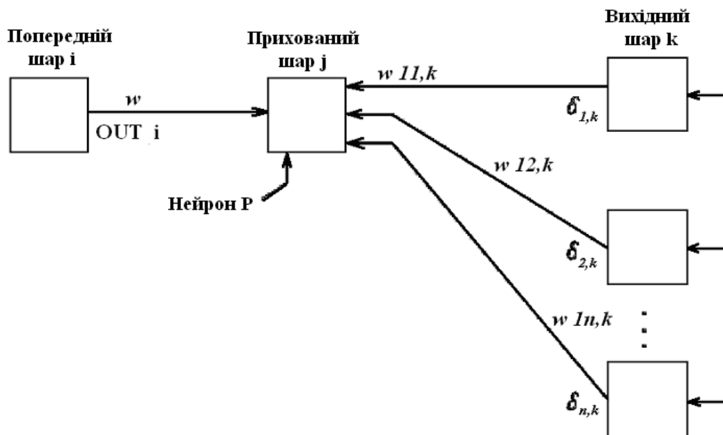
Рис. 3.9 – Підстроювання ваг прихованого шару
