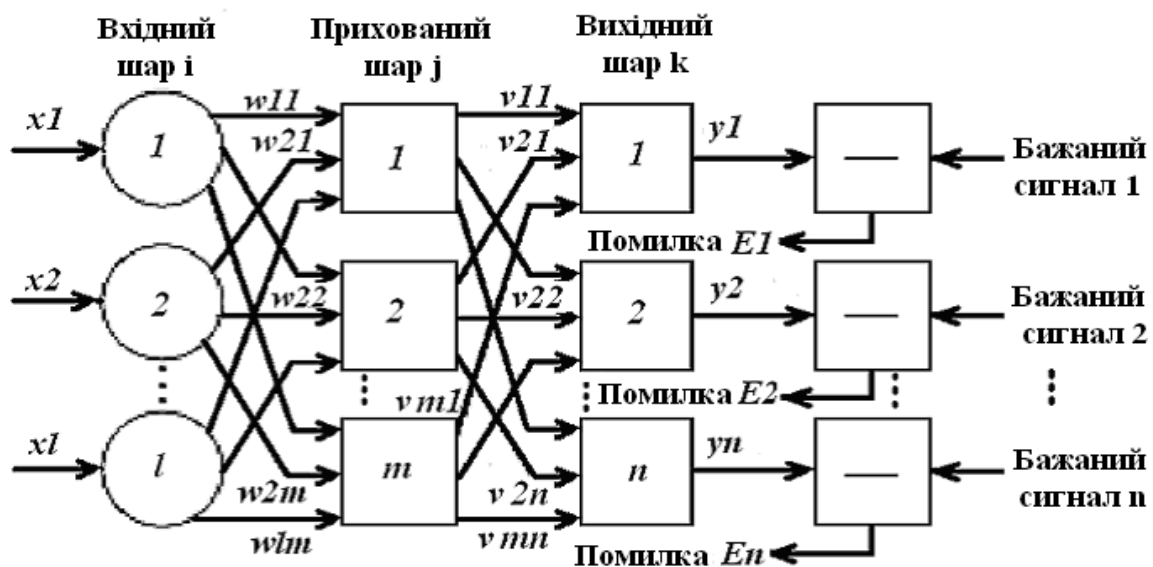
Рис. 3.7 – Процедура навчання багатошарового персептрона
