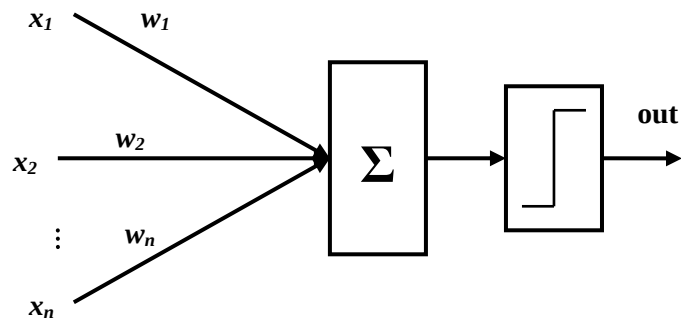
Рис. 3.1 – Персептронний нейрон Уоррена Мак-Каллока і Вальтера Піттса
