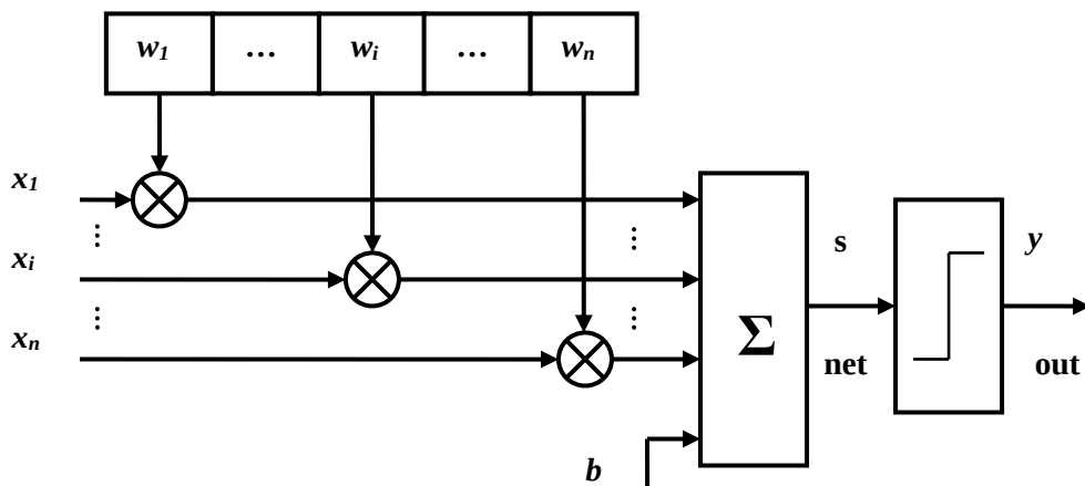
Рис. 3.2 – Структурна схема одношарового персептрона з одним виходом
