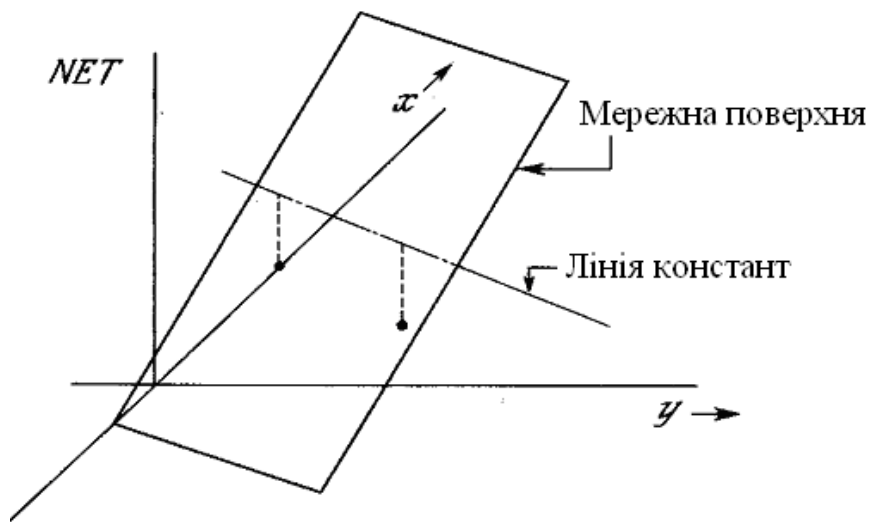
Рис. 3.5 – Персептронна NET-площина
