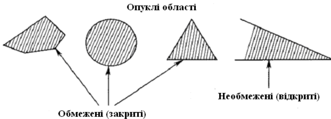
Рис. 3.10 – Опуклі обмежені і необмежені області
