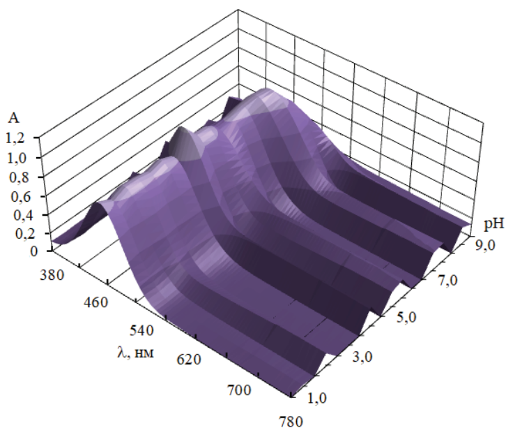
Рис. 6. Залежність спектрів поглинання системи \text{H}_2\text{SO}_4 - \text{MEA} - \text{TrOOO} - \text{H}_2\text{O} від pH середовища.
