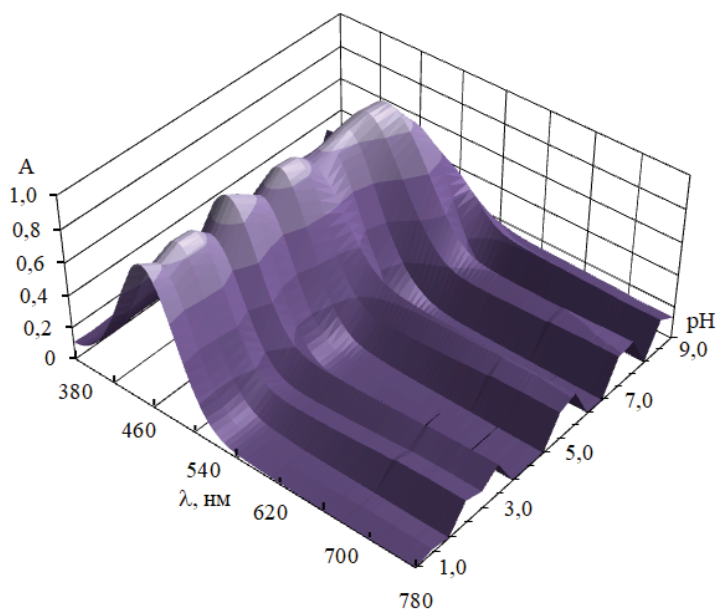
Рис. 5. Залежність спектрів поглинання системи \text{HClO}_4 - \text{MEA} - \text{TrOOO} - \text{H}_2\text{O} від pH середовища.
