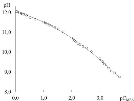
Рис. 1. Концентраційна залежність pH водних розчинів MEA при 293 К.
