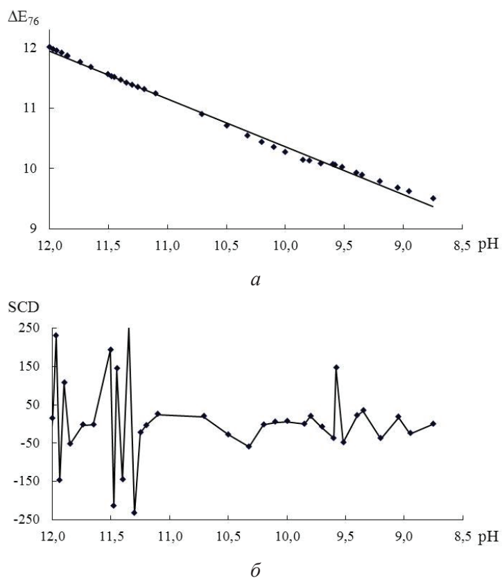
Рис. 3. Залежності величин кольориметричних функцій \Delta E_{76} (а) та \text{SCD} (б) системи \text{MEA} - \text{TrOOO} - \text{H}_2\text{O} в від \text{pH} середовища.
