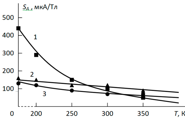
Рис. 5. Залежність магніточутливості ДМТС від температури для різних матеріалів 1 – високоомний кремній, 2 – низькоомний кремній, 3 епітаксialна плівка
