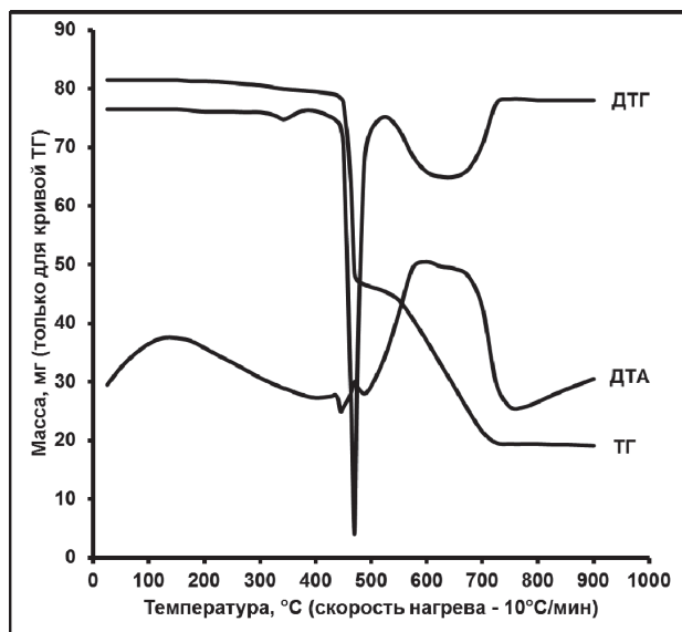
Рис. 1. Термогравиграмма комплекса [\text{Sn}(\text{Bnf})_2] (V).
