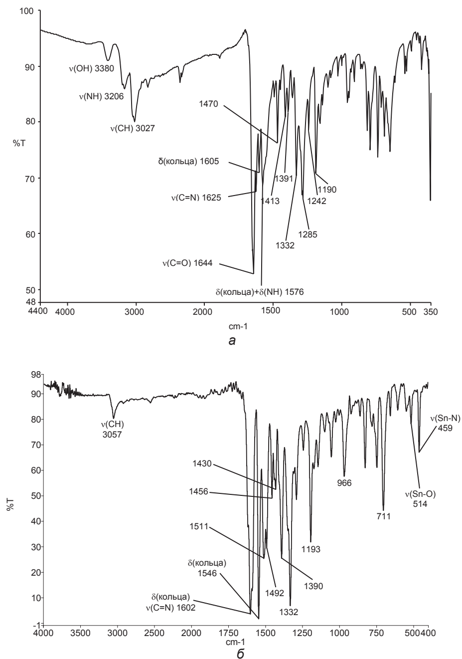
Рис. 2. ИК-спектры H_2Bnf (а) и [Sn(Bnf)_2] (V) (б).
