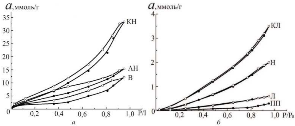
Рис. 1. Изотермы сорбции паров воды ВН ●- сорбция, ○- десорбция
