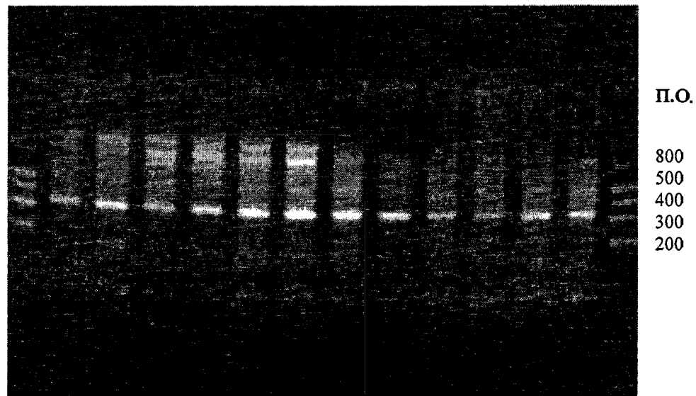
Рис. 1. Електрофорез продуктів ПЛР в агарозному гелі. 1, 2 — T_{від} = 53^\circ C , 1,3 мМ Mg^{++} ; 3, 4 — T_{від} = 53^\circ C , 1,7 мМ Mg^{++} ; 5, 6 — T_{від} = 53^\circ C , 2,0 мМ Mg^{++} ; 7, 8 — T_{від} = 61^\circ C , 1,3 мМ Mg^{++} ; 9, 10 — T_{від} = 61^\circ C , 1,7 мМ Mg^{++} ; 11, 12 — T_{від} = 61^\circ C , 2,0 мМ Mg^{++} ; М — маркери молекулярної ваги.
