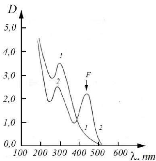
Fig.3.12. Absorption spectra of crystal NaCl: MnCl_2 \cdot 4H_2O .
