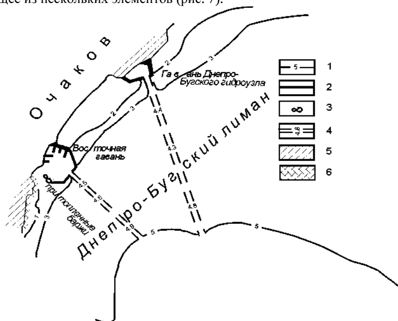
Рис. 6. Расположение различных положительных и отрицательных искусственных форм рельефа в западной части Днепро-Бугского лимана, северное побережье Черного моря. Обозначения: 1 — изобаты (в м); 2 — искусственные сооружения (молы, пирсы, причалы, валы, гряды); 3 — притопленные баржи; 4 — судоходный канал с отметками глубин (в м); 5 — искусственные песчаные насыпи; 6 — защитная каменная наброска.
