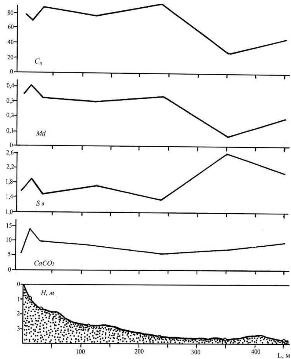
Рис. 4. Типичный поперечный профиль подводного склона моря на участке сопряжения абразионного берега и корня Лагерной косы, и распределение на нем основных свойств наносов: C_0 — ведущая фракция, %%; Md — медианный диаметр, мм; S_0 — коэффициент сортировки; CaCO_3 — содержание карбонатного материала, %%.
