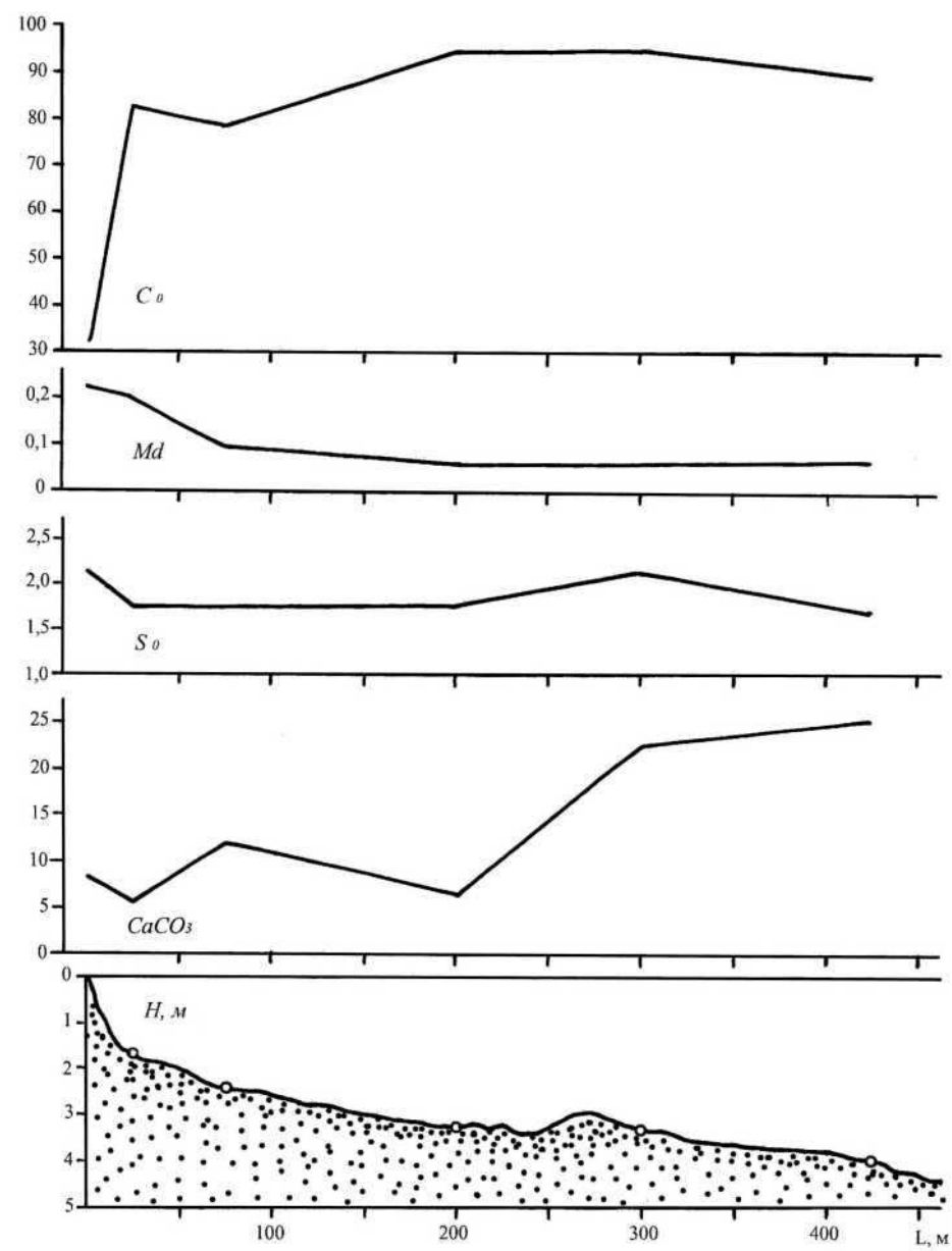
Рис. 3. Типичный поперечный профиль подводного склона моря на участке западнее сооружений морского порта и распределение на нем основных свойств наносов: C_0 — ведущая фракция, %%; Md — медианный диаметр, мм; S_0 — коэффициент сортировки; CaCO_3 — содержание карбонатного материала, %%.
