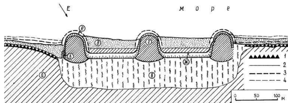
Рис. 7. Берегозащитное и противооползневое гидротехническое сооружение на участке санатория «Очаков» к западу от причалов порта Очаков. Условные обозначения: 1 — линия активного клифа после строительства сооружения; 2 — береговая линия пляжа после строительства сооружения; 3 — линия активного клифа до строительства сооружения; 4 — береговая линия пляжа до строительства сооружения. Элементы сооружения: а — поверхность коренного глинистого берега; б — искусственный откос после выполаживания склона; в — каменная наброска на наветренном входящем углу; г — искусственный бетонный выступ с мористым пологим откосом для гашения волн («фигурная берма»); д — песчаный пляж; е — пологий откос во фронтальной части бетонного выступа. Е — результирующий энергетический вектор ветро-волнового режима.
