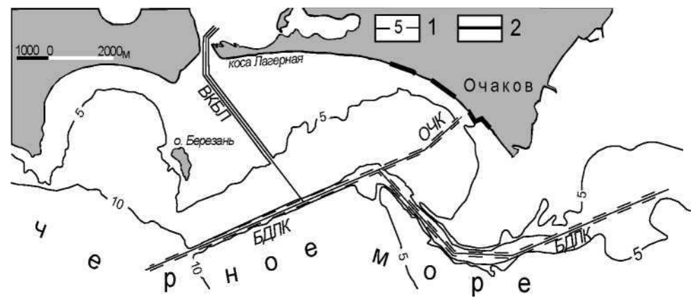
Рис. 5. Расположение искусственных отрицательных форм донного рельефа — судоходных каналов на дне северной части Черного моря. Обозначения: 1 — изобаты (в м); 2 — береговые искусственные гидротехнические сооружения; БДЛК — Бугско-Днепровский лиманский канал; ВКБЛ — входной канал Березанского лимана; ОЧК — Очаковский судоходный канал.
