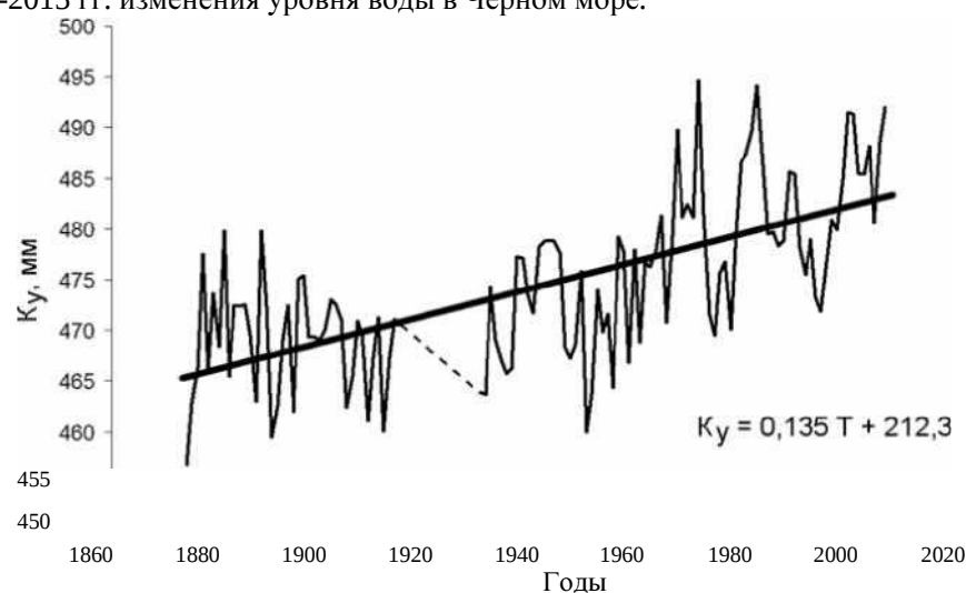
Рис. 8. График изменения средних годовых значений уровня Черного моря на гидрометеорологической станции «Очаков» в период 1870—2007гг.
