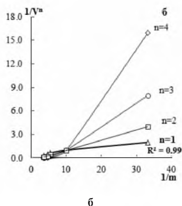
Рис. 2. Определение состава комплексов \text{Bi(III)} с ДФДОХ методом прямой линии Асмуса: (а) комплекс при рН 1,9 ( \lambda=510 нм); (б) комплекс при рН 4,6 ( \lambda=550 нм); C_{\text{Bi}}=1 \cdot 10^{-5} М, C_{\text{ДФДОХ}}=4 \cdot 10^{-5} М; 0,08% поливинилового спирта; l=1 см
