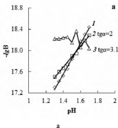
Рис. 3. Зависимость степени закомплексованности от кислотности среды: (а) pH 1–2; (б) pH 4–5; 1 — Bi^{3+} ; 2 — BiOH^{2+} ; 3 — Bi(OH)_2^+
