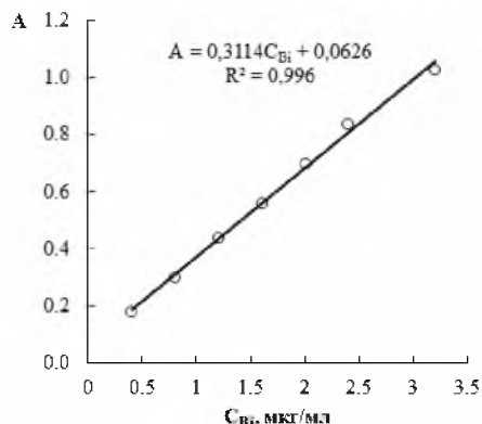
Рис. 4. Градуировочный график для определения Bi(III) с ДФДОХ: l=2 см, \lambda=510 нм, 0,08 поливинилового спирта, pH 1,9
