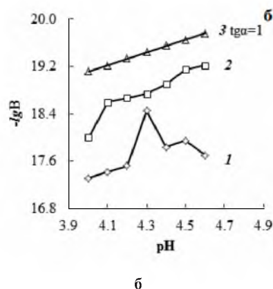
Рис. 3. Зависимость степени закомплексованности от кислотности среды: (а) pH 1–2; (б) pH 4–5; 1 — Bi^{3+} ; 2 — BiOH^{2+} ; 3 — Bi(OH)_2^+
