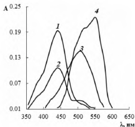
Рис. 1. Спектры светопоглощения в системе « \text{Bi(III)} –ДФДОХ»: 1, 2 – реагент при рН 1,9 и рН 4,6 соответственно (раствор сравнения – дистиллированная вода); 3 – комплекс при рН 1,9; 4 – комплекс при рН 4,6 (раствор сравнения – «холостой опыт»); C_{\text{Bi(III)}}=1 \cdot 10^{-5} М; C_{\text{ДФДОХ}}=4 \cdot 10^{-5} М; 0,08% поливинилового спирта; l=1 см
