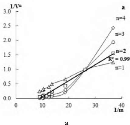
Рис. 2. Определение состава комплексов \text{Bi(III)} с ДФДОХ методом прямой линии Асмуса: (а) комплекс при рН 1,9 ( \lambda=510 нм); (б) комплекс при рН 4,6 ( \lambda=550 нм); C_{\text{Bi}}=1 \cdot 10^{-5} М, C_{\text{ДФДОХ}}=4 \cdot 10^{-5} М; 0,08% поливинилового спирта; l=1 см
