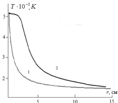
Рис. 2. Температурные профили расширяющейся плазмы с центральным источником: 1 – расчет по аналитическому решению, 2 – расчет методом численного интегрирования с интенсивно идущими рекомбинационными и ионизационными процессами
