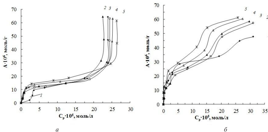
Рис. 2. Ізотерми сорбції КО аніоном Граніон АВА-Г1, які отримані при pH 5 (а) та pH 9 (б) при різних температурах Т, К: 1 – 293; 2 – 298; 3 – 303; 4 – 308; 5 – 313.
