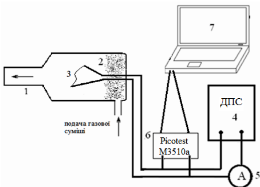
Рис. 1. Первинний пристрій: 1 – колба, 2 – поруватий матеріал, 3 – платинова нитка, 4 – джерело постійного струму Б5-47, 5 – амперметр М890Г, 6 – мультиметр Picotest M3510a, 7 – комп'ютер
