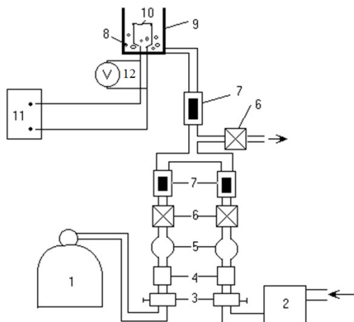
Рис. 3. Експериментальна установка: 1 – балон з воднем, 2 – повітряний компресор, 3 – редуктори, 4 – фільтри, 5 – фільтри Шота, 6 – крани, 7 – ротаметри, 8 – на-сипка, 9 – реакційний посуд, 10 – платинова нитка, 11 – джерело постійного струму Б5-47, 12 – мультівольметр Picotest M3510A.
