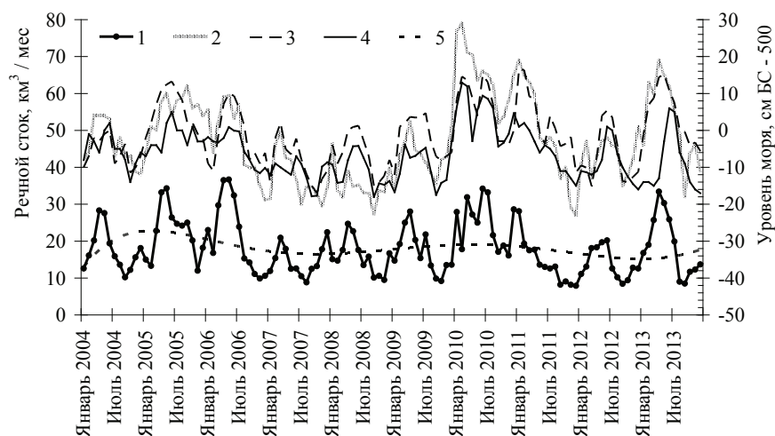
Рис. 2. Среднеемесячные значения стока р. Дунай (1) с аппроксимацией полиномом 6-й степени (5) и уровня моря на ГМС «Приморское» (2), НИС «О. Змеиный» (3) и ГМС «Черноморское» (4) в 2004-2013 гг.
