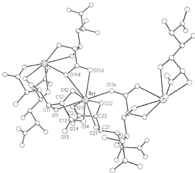
Рис. 5. Кристаллическая структура галактарата стронция [15]
