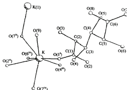
Рис. 7. Структура \text{HOOC}(\text{CHOH})_4\text{COOK} [17]
