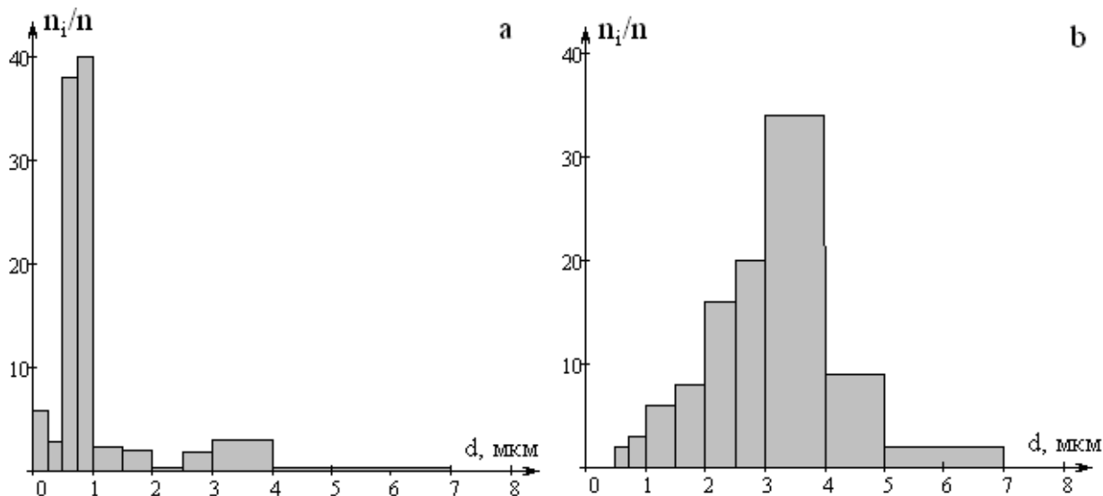
Рис. 1 Распределение по размеру (эквивалентному диаметру) а) частиц окиси кремния, полученного в кипящем слое и б) частиц нашатыря, полученных возгонкой в камере.
