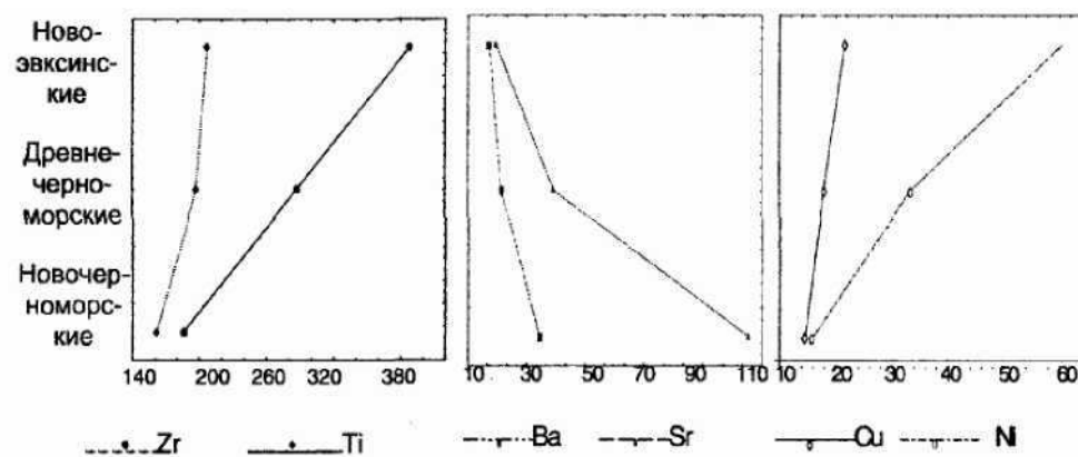
Рис.2. Содержание элементов в толще голоценовых отложений. Содержание Ti, Ba, Sr, n \cdot 10^{-3} \% , Zr, Cu, Ni, n \cdot 10^{-4} \%
