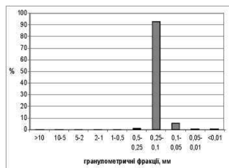
Рис. 4. Гістограма розподілу гранулометричних фракцій у приурізових відкладах Анкудінова гирла поблизу „0-й кілометр”
