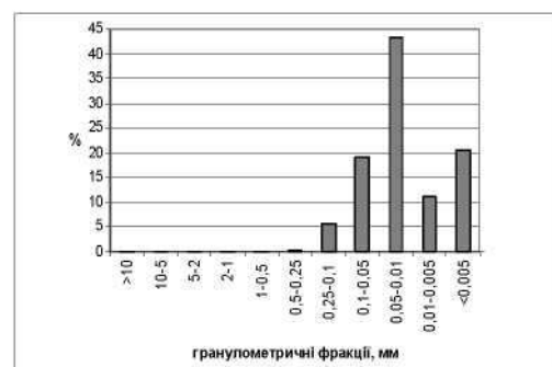
Рис. 3. Гістограма розподілу гранулометричних фракцій у відвалах днозаглиблення в м. Вилкове.
