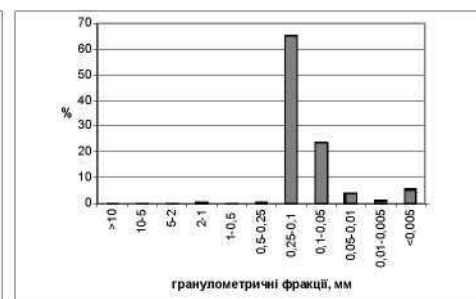
Рис. 6. Гістограма розподілу гранулометричних фракцій в дрібнозернистих пісках узмор'я гирла Бистре
