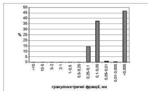
Рис. 5. Гістограма розподілу гранулометричних фракцій в крупноалевритістих пелітах узмор'я гирла Бистре
