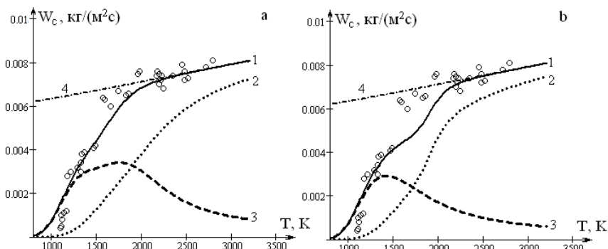
Рис. 3. Температурные зависимости скоростей химических реакций (1 – W_C , 2 – W_{C,s} , 3 – W_{C,v} , 4 – W_{Cd} ) пористой частицы графита ЭГ-14 ( d = 15 мкм) в ламинарном воздушном потоке ( w = 0.6 м/с): а) учет и б) без учета эндотермической реакции (III) внутри пор. о – эксперимент Головиной [4].
