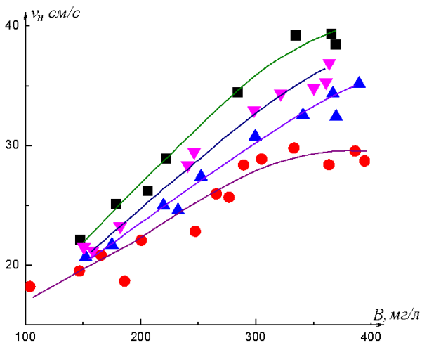
Рис.1. Зависимость нормальной скорости пламени от концентрации горючего в двухкомпонентной газовой смеси Al – Zr. ■ – 100% Zr; ▼ – 50% Al + 50% Zr; ▲ – 25% Zr + 75% Al; ● – 100% Al.
