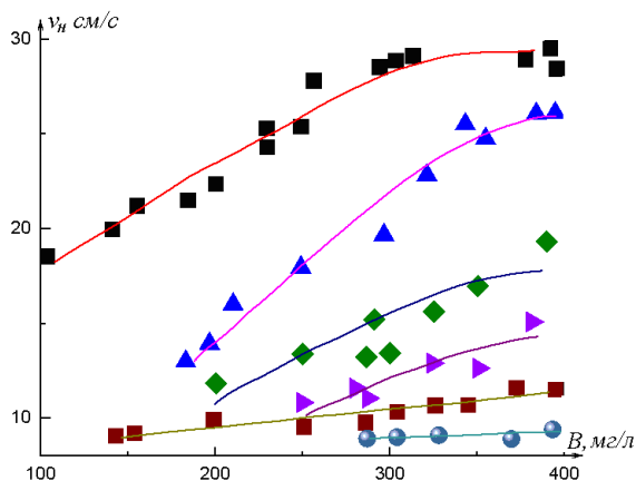
Рис.3. Зависимость нормальной скорости пламени от концентрации горючего в двухкомпонентной газозвеси Al-Fe . ■ – 100% Al ; ▲ – 75% Al + 25% Fe ; ◆ – 50% Fe + 50% Al ; ● – 100% Fe ; ◆ – 90% Fe + 10% Al .
