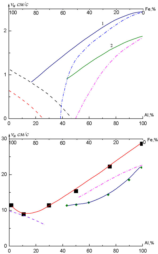
Рис. 4. Зависимость нормальной скорости пламени от состава двухкомпонентной газовой смеси Al/Fe а – расчет; б – эксперимент; 1 – V = 300 мг/л; 2 – V = 200 мг/л; - - - - Al / инертное в-во; - - - - Fe / инертное в-во.
