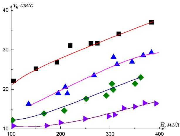
Рис.2. Зависимость нормальной скорости пламени от концентрации горючего в двухкомпонентной газовой смеси Al – Mg. ■ – 100% Mg; ▼ – 50% Al + 50% Mg; ◆ – 25% Mg + 75% Al; ► – 100% Al.
