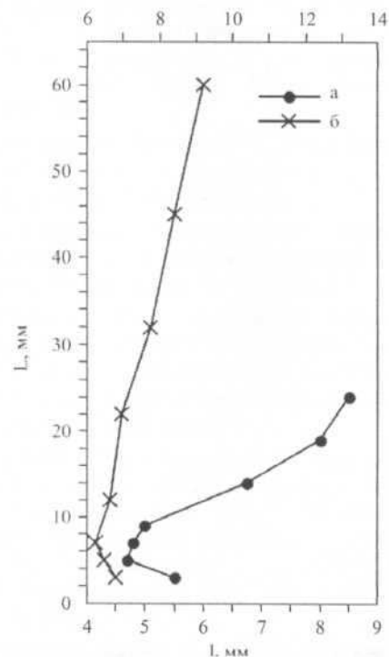
Рис. 6. Вертикальные распределения местоположения вдоль оси симметрии факела минимумов величин напряжений электрического пробоя факела в зависимости от их положения в горизонтальных распределениях. a – стехиометрическое соотношение; b – обогащённая смесь.
