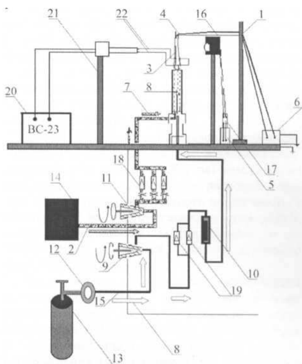
Рис. 1. Схема экспериментальной установки: 1, 21 – препаратоводители; 2, 15 – трубопроводы; 3 – исследуемое пламя; 4 – спай термопары, находящийся в исследуемом пламени; 5 – осциллограф С1-112А; 6 – вольтметр В7-35; 7 – направление движения воздуха; 8 – направление движения газа; 9 и 11 – игольчатые краны; 10 – пламегаситель (стружки металла); 12 – редуктор грубой регулировки давления газа; 13 – газовый баллон; 14 – компрессор; 16 – фотодиод; 17 – усилитель; 18 – блок ротаметров, измеряющий расход воздуха; 19 – блок ротаметров, измеряющий расход газа; 20 – источник высокого напряжения ВС-23; 22 – электроды.
