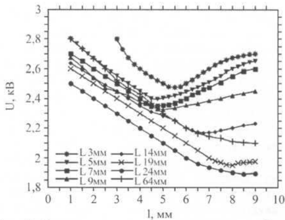
Рис. 3. Распределение величин напряжения пробоя в горизонтальном сечении факела для смеси стехиометрического состава (изображение факела, рис. 2а).
