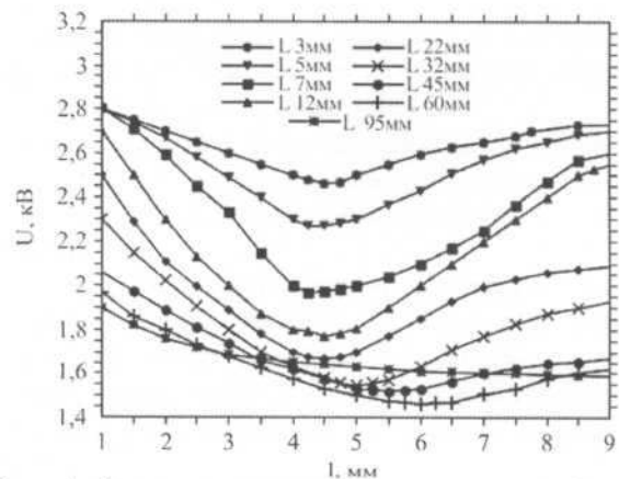
Рис. 4. Распределение величин напряжения пробоя в горизонтальном сечении факела для обогащённой смеси (изображение факела, рис. 2б).
