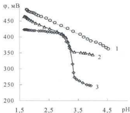
Рис. 5. Зависимость потенциала платинового электрода от pH водных растворов тетрафтороборной кислоты ( C_{\text{HBF}_4}^0 = 0,02 \text{ М} (1); 0,20 \text{ М} (2); 0,40 \text{ М} (3)) в процессе титрования их водными растворами ГМТА ( C_{\text{ГМТА}}^0 = 0,10 \text{ М} (1); 1,00 \text{ М} (2, 3)).
