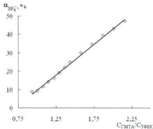
Рис. 4. Зависимость степени гидролиза тетрафтороборат-иона от соотношения C_{\text{GMTA}}/C_{\text{ТФБК}} при титровании 0,02 М раствора \text{HBF}_4 0,10 М раствором ГМТА.
