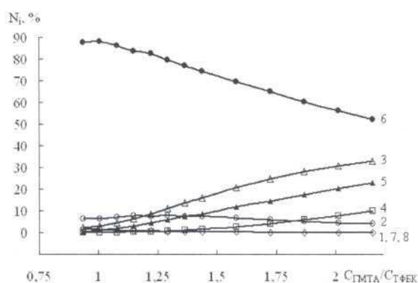
Рис. 3. Диаграммы частичного распределения ион-молекулярных форм в системе «Н 2 О – ТФБК – ГМТА» в зависимости от соотношения C_{ГМТА}/C_{ТФБК} при 20 °С. N_i – мольная доля BF_4^-(1) ; BF_3OH^-(2) ; BF_2(OH)_2^-(3) ; BF(OH)_3^-(4) ; фторидных комплексов ( I_{МК} + I_{ИК} ) (5) и ионной пары ( II_{ИП} ) (6); F^- (7); HF (8) относительно общего бора (1–6) и фтора (7, 8).
