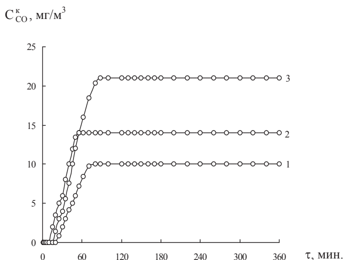
Рис. Изменение C CO K во времени при окислении СО кислородом в присутствии Pd/Al 2 O 3 – катализатора при разных C CO H в ГВС C CO H , мг/м 3 : 1 – 100; 2 – 200; 3 – 300; ω = 1,67×10 -2 л/с; d 3 = 1-2 мм; T = 293 К; φ ГВС = 70 %; m k = 4 г; t' = 0,42 с; U = 5,3см/с.
