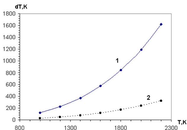
Рис.3. Разность между локальной температурой газа и температурой нити в зависимости от температуры нити: 1) d = 100 мкм; 2) d = 20 мкм ( \varepsilon = 0,7 ).
