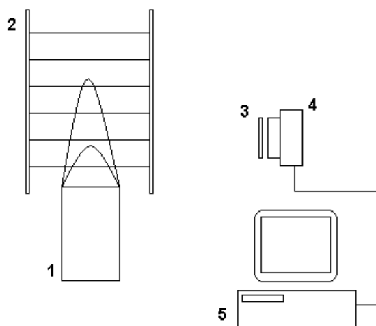
Рис. 1. Схема экспериментальной установки: 1 – горелка Бунзена; 2 – касета с кварцевыми нитями; 3 – интерференционный фильтр; 4 – цифровая камера; 5 – компьютер.
