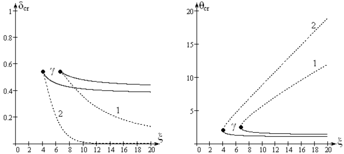
Рис. 3. Зависимость критических значений безразмерного диаметра \delta_{i,e} (а) и температуры \theta_{i,e} (б) от параметра \xi при \gamma_g = 0.1 :
