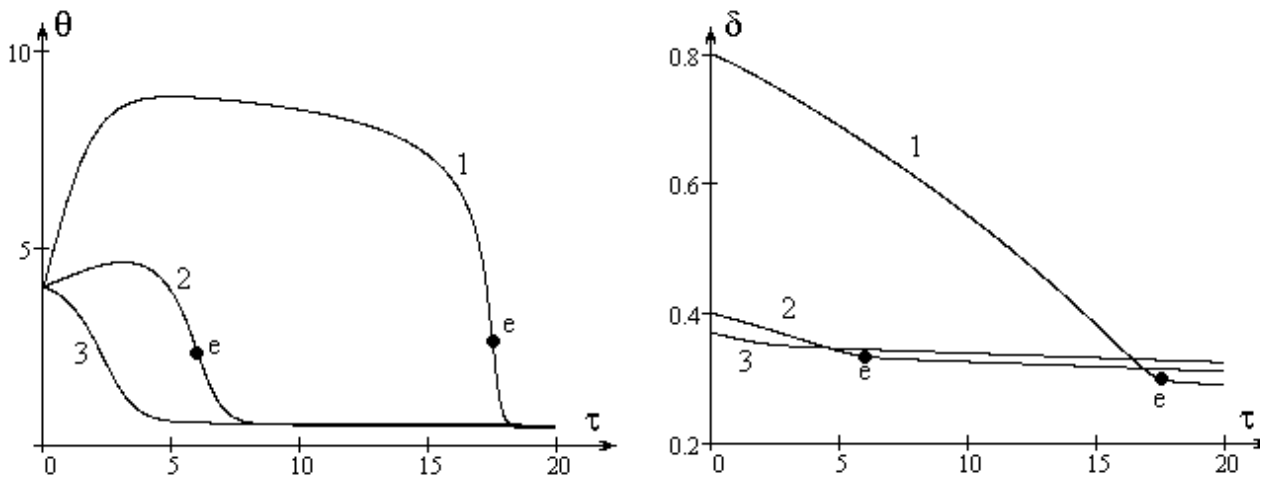
Рис. 5. Временные зависимости безразмерной температуры \theta и диаметра \delta при \theta_b = 4 , \xi = 10 , \gamma_g = 0.1 , \gamma_c = 0.025 . 1) \delta_b = 0.8 , 2) \delta_b = 0.4 , 3) \delta_b = 0.37 .
