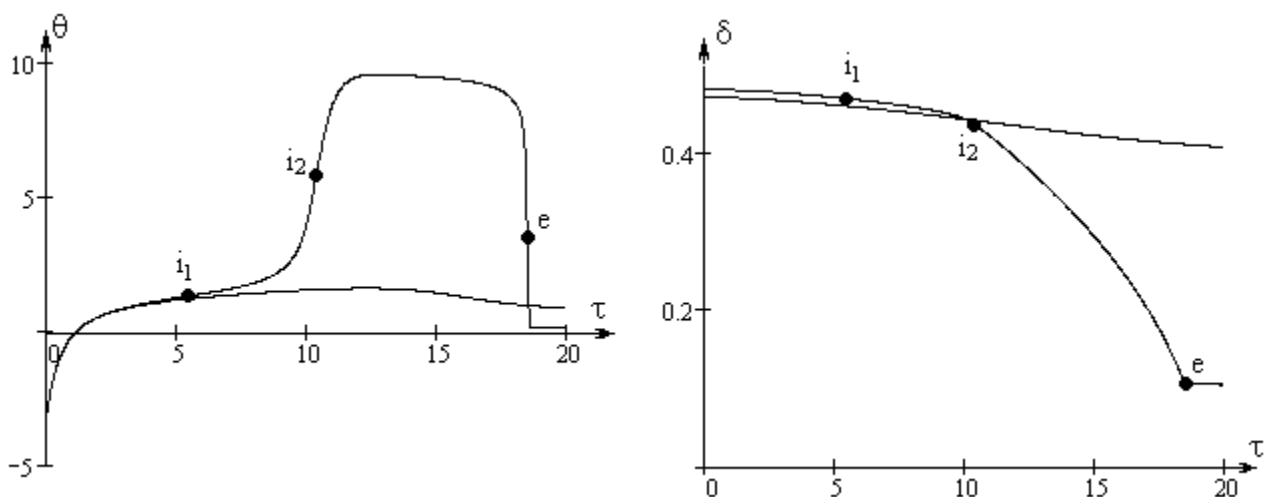
Рис. 6. Временные зависимости безразмерной температуры \theta и диаметра \delta при \theta_b = -3 , \xi = 10 , \gamma_g = 0.05 , \gamma_c = 0.025 . 1) \delta_b = 0.48 , 2) \delta_b = 0.47 .
