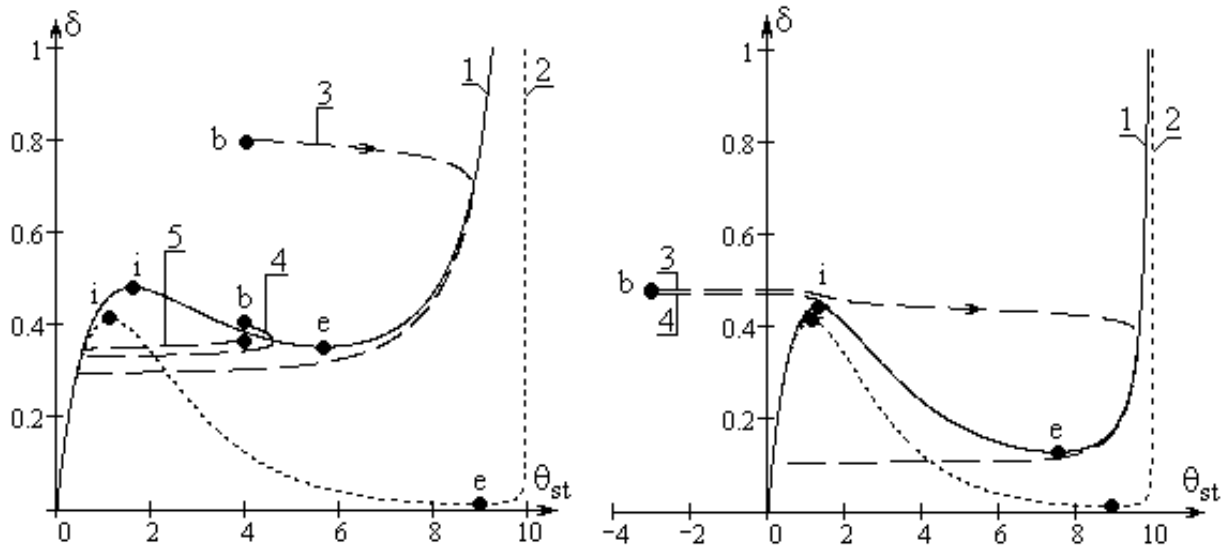
Рис. 2. Зависимость безразмерного диаметра от стационарной температуры \delta(\theta) , найденная по формуле (5) (сплошная, кривая 1) и (6) (пунктир, кривая 2) при \xi = 10 , а) \gamma_g = 0.1, \gamma_Q = 0.1 ; б) \gamma_g = 0.05, \gamma_Q = 0.025 .
