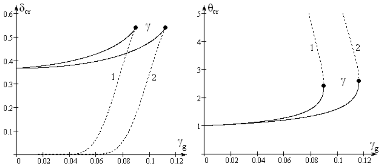
Рис. 4. Зависимость критических значений безразмерного диаметра \delta_{i,e} (а) и температуры \theta_{i,e} (б) от безразмерной температуры газа \gamma_g при \gamma_Q = 0.5 :
