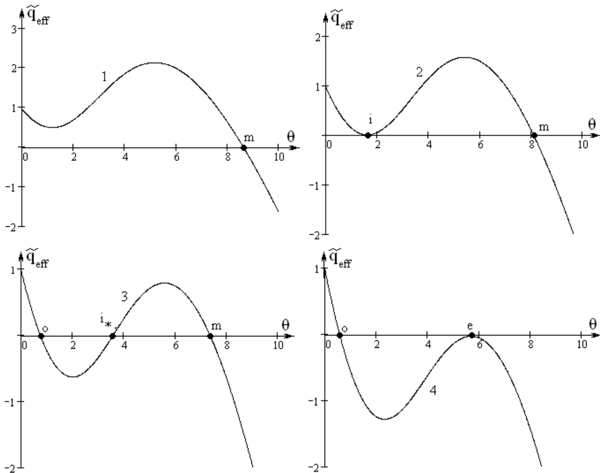
Рис. 1. Зависимость эффективной плотности тепловыделения от температуры \tilde{q}_{eff}(\theta) при \xi = 10, \gamma_g = 0.1 ; 1) \delta = 0.60 ; 2) \delta = 0.48 ; 3) \delta = 0.40 ; 4) \delta = 0.35 .
