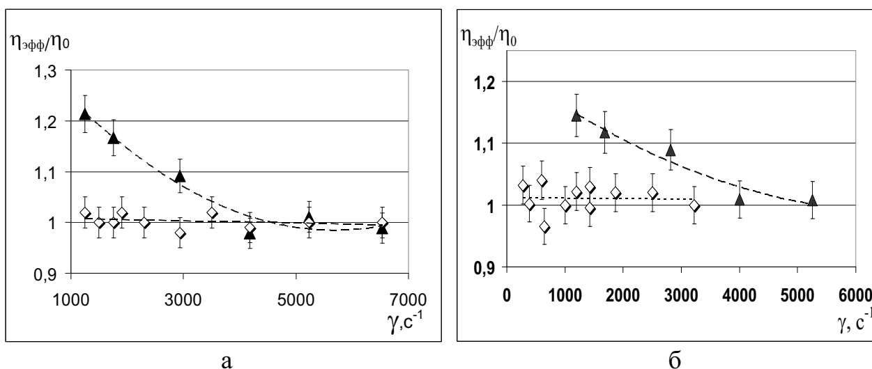
Рис.1. Зависимость относительной вязкости микронных прослоек заводских синтетических масел от приложенных скоростей деформаций: а – масло SAE 5W40, б – масло BP 180. Толщина прослоек D : ▲ – 1.5 мкм; ◇ – 4.5÷50 мкм. T = 295 \div 297 К.
