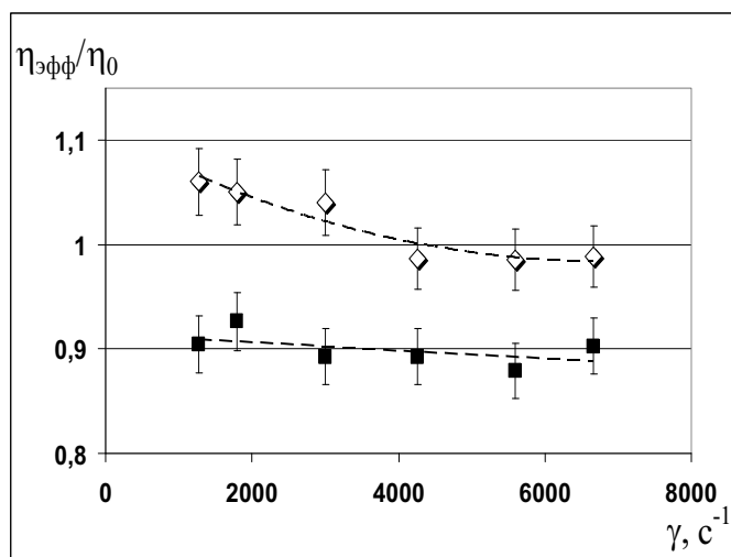
Рис. 3. Зависимость относительной вязкости микронных прослоек толщиной D \approx 1.5 мкм синтетических масел с добавкой воды ( C_{об} \approx 5\% ) от приложенных скоростей деформаций: \diamond - масло BP 180; \blacksquare – масло SAE 5W40. T = 292 \div 300 K.
