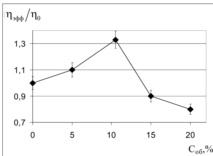
Рис. 4. Зависимость коэффициента относительной вязкости прослойки толщиной D \approx 1.5 мкм синтетического масла на основе полигликоля от объемной концентрации добавленной воды. T = 292 \div 298 K.
