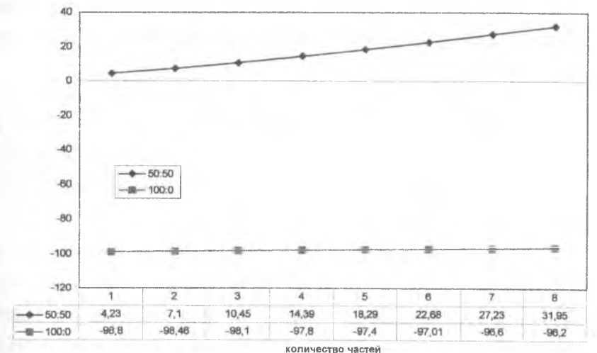
Рис. 2.4. График зависимости относительной структурной дисгармонии от количества градаций для различных соотношений частей в модуле
