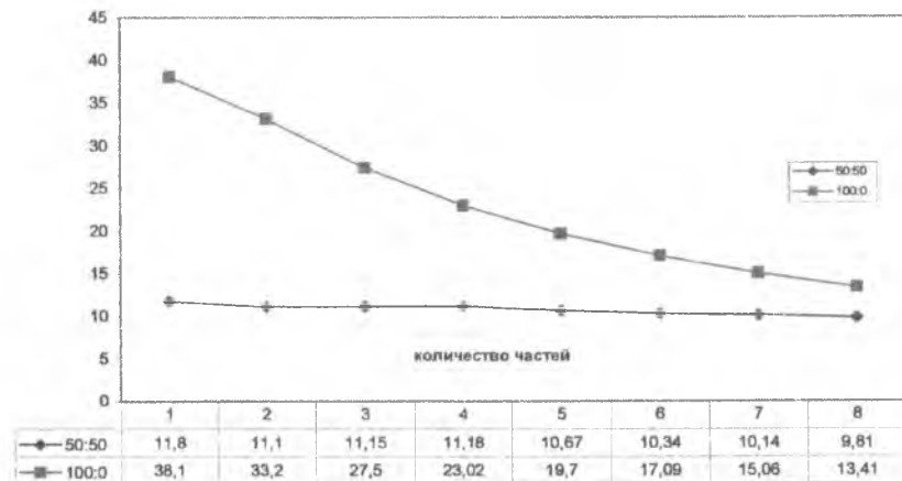
Рис. 2.3. График зависимости абсолютной структурной дисгармонии от количества частей для различных соотношений между частями в модуле (50:50 и 100:0)
