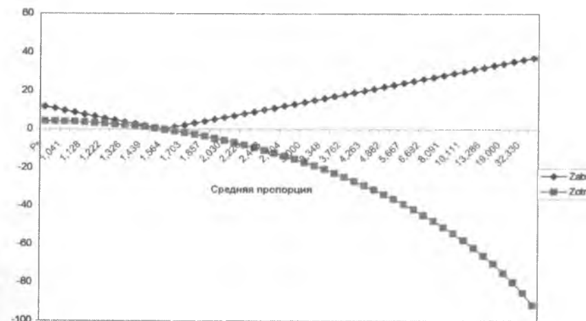
Рис. 2.2. Зависимость абсолютной структурной и относительной дисгармонии от средней пропорции для социального модуля, состоящего из 2-х частей
